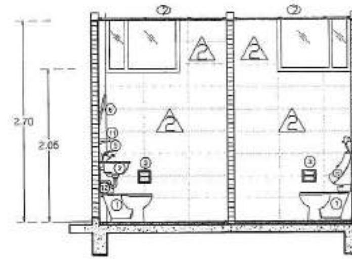
รูปตัดขยาย 1-B มาตราส่วน 1 : 50
