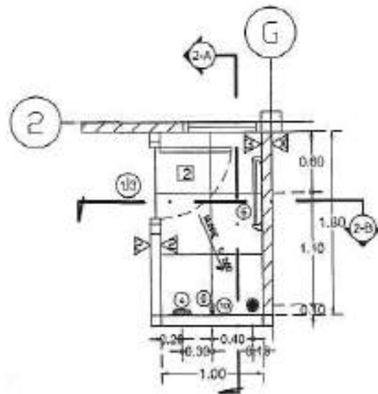
แบบขยายห้องชักล้าง มาตราส่วน 1 : 50
