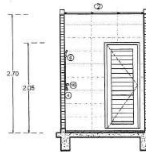
รูปตัดขยาย 2-A มาตราส่วน 1 : 50
