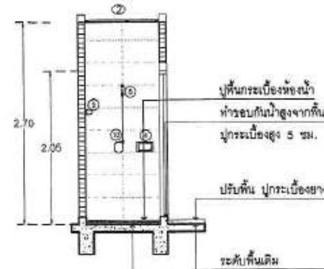
รูปตัดขยาย 2-B มาตราส่วน 1 : 50
