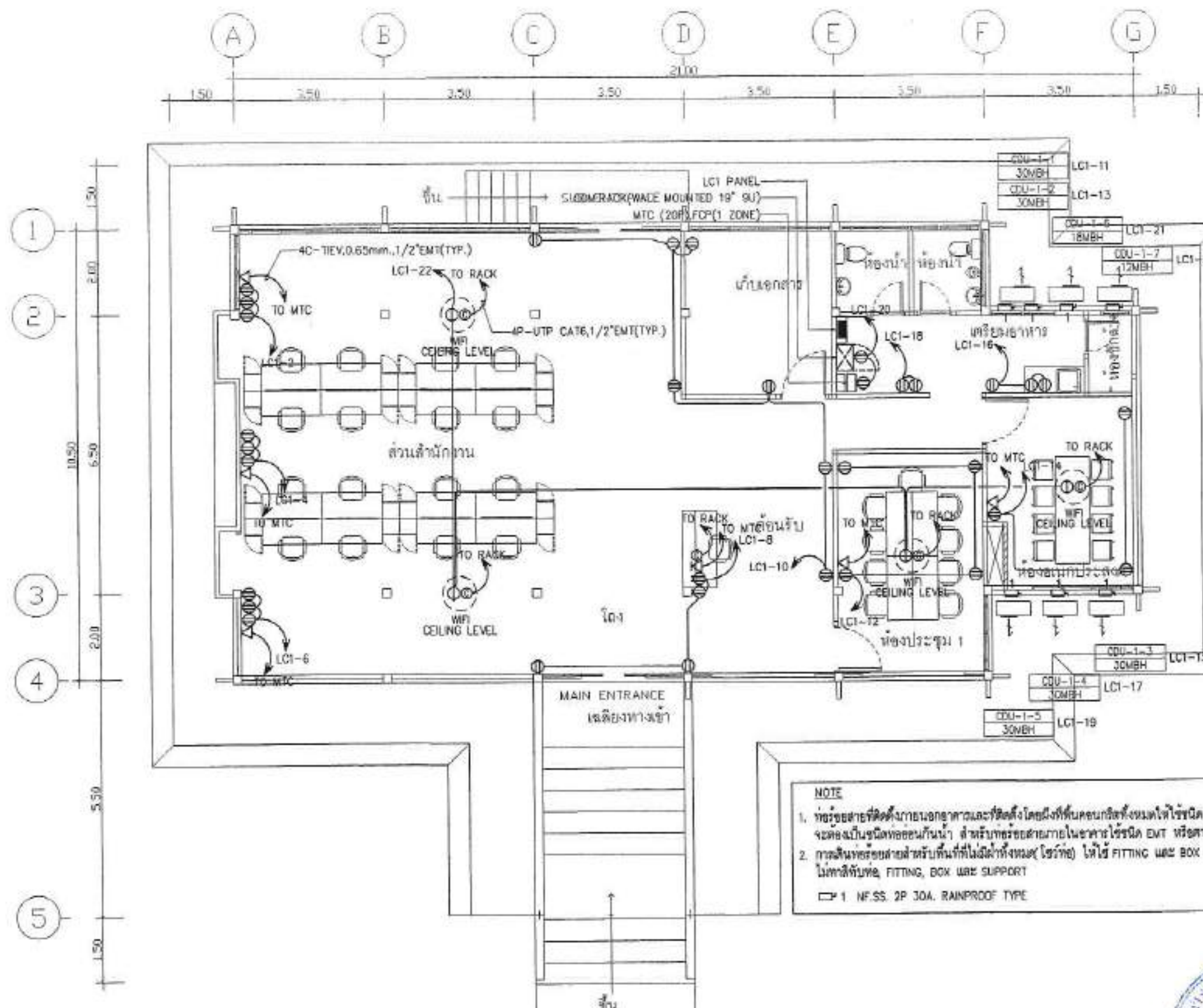
แปลนตัวรับไฟฟ้า, โทรศัพท์และคอมพิวเตอร์ ชั้นที่ 1 (ห้องประชุม) มาตราส่วน 1:100
