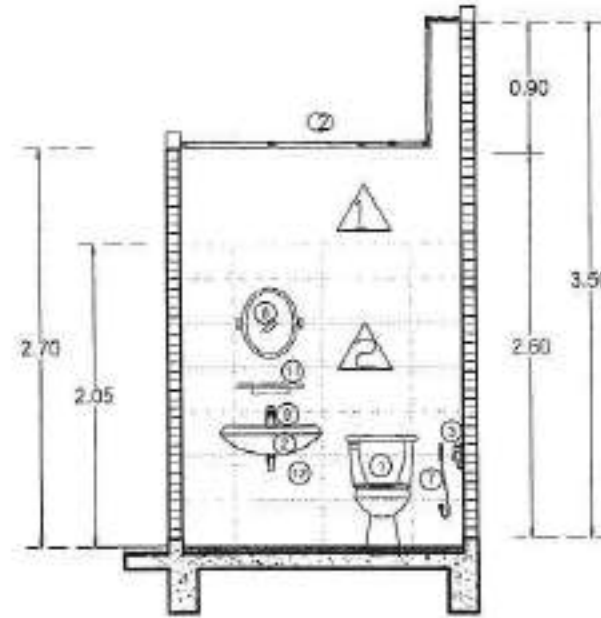
รูปตัดขยาย 1-A มาตราส่วน 1 : 50
